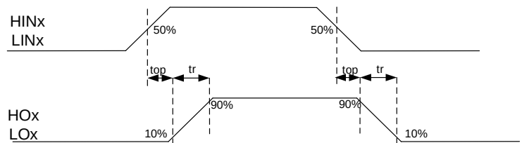
图 5-4 开关时间
