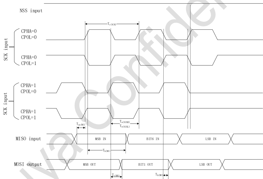
图 5-3 SPI 时序图 – 主机模式
