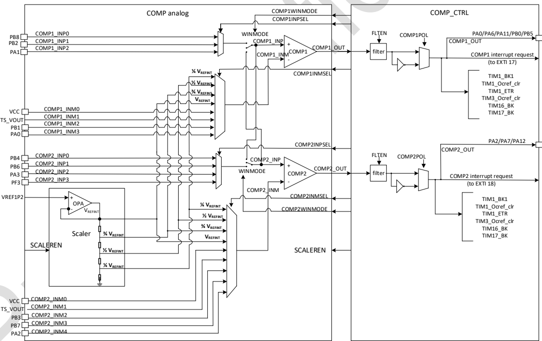
图 2-5 COMP 框图
