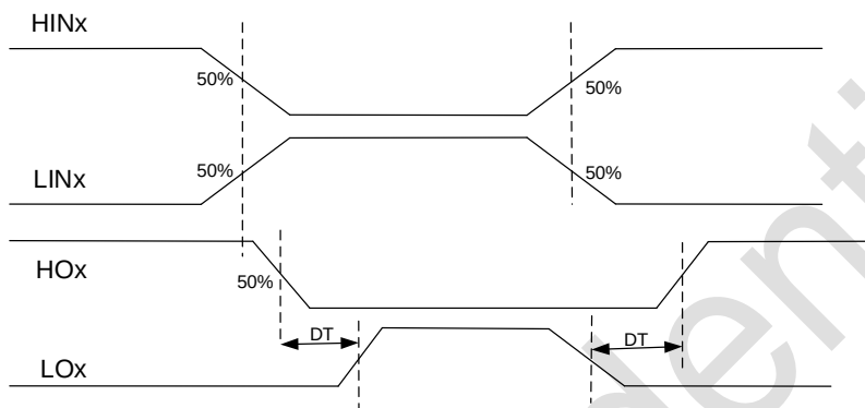
图 5-6 死区功能
