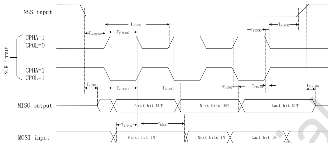
图 5-2 SPI 时序图 – 从机模式, CPHA=1
