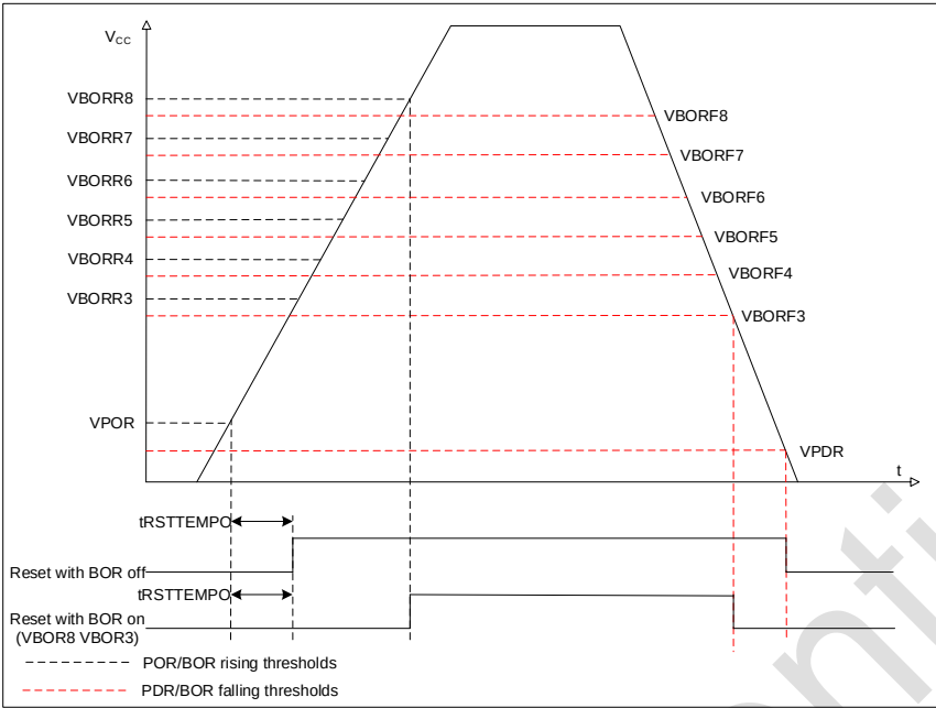
图 2-3 POR/PDR/BOR 阈值
