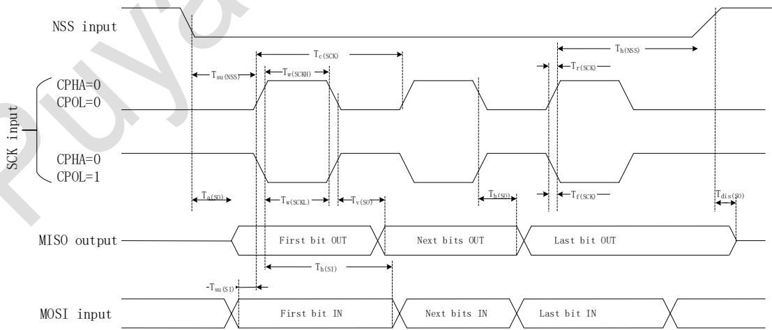
图 5-1 SPI 时序图 – 从机模式，CPHA=0
