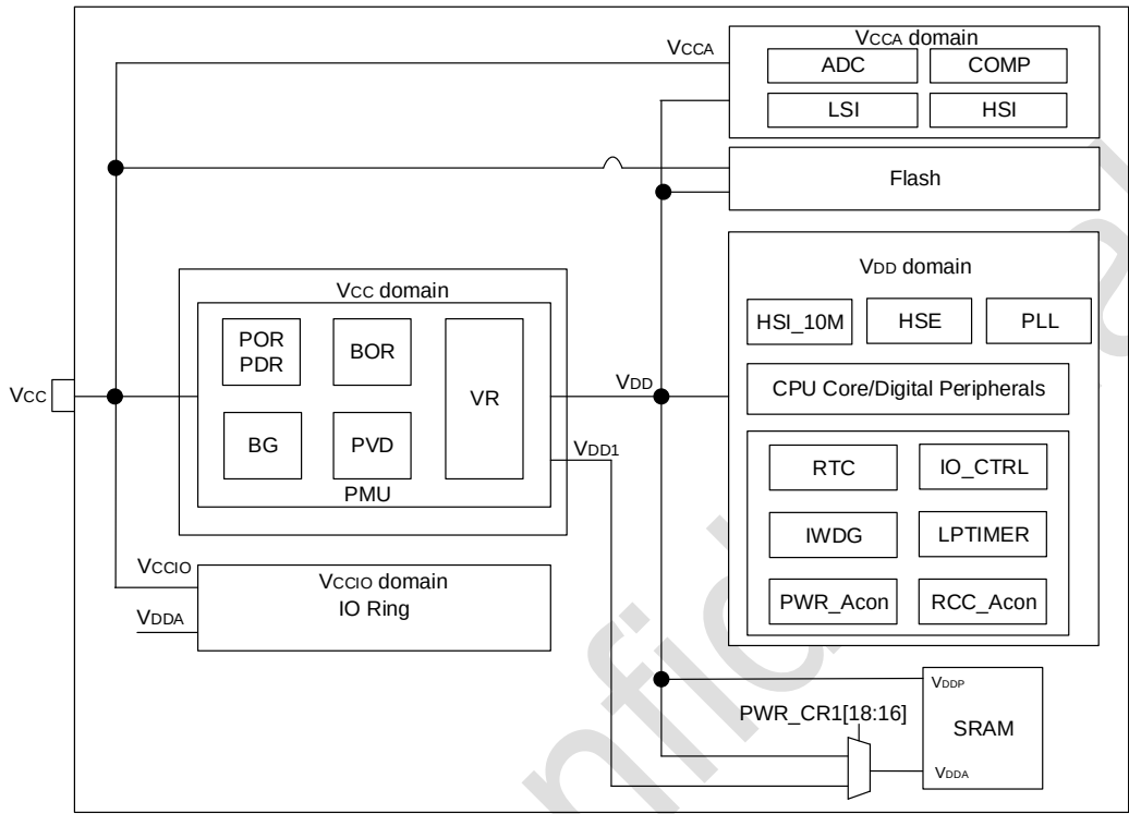
图 2-2 电源框图
